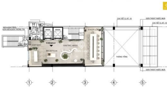
Sơ đồ mặt bằng MK Center Premium
