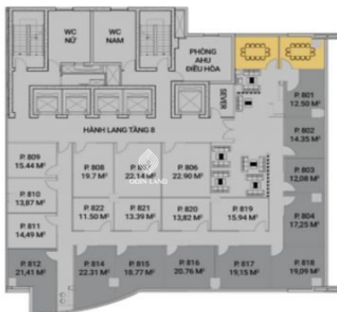
Sơ đồ mặt bằng MPro Phạm Hùng
