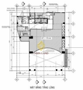
Mặt bằng tầng lửng
