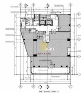
Mặt bằng tầng 13
