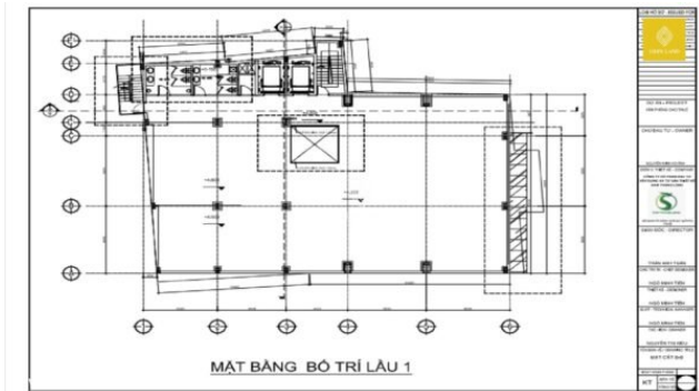
Thiết kế sàn 1 tòa nhà
