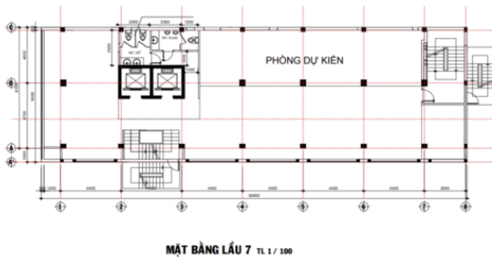
Sơ đồ mặt bằng
