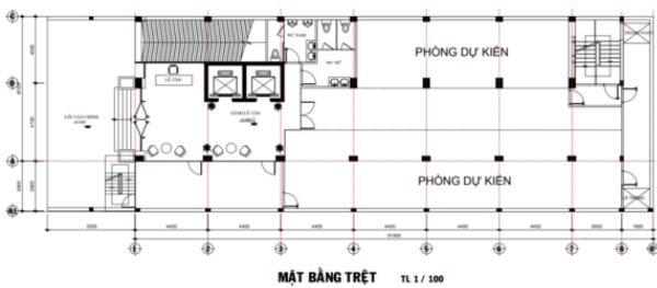
Sơ đồ mặt bằng
