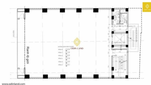
Mặt bằng tầng 3-8
