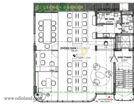
Sơ đồ mặt bằng tầng 2
