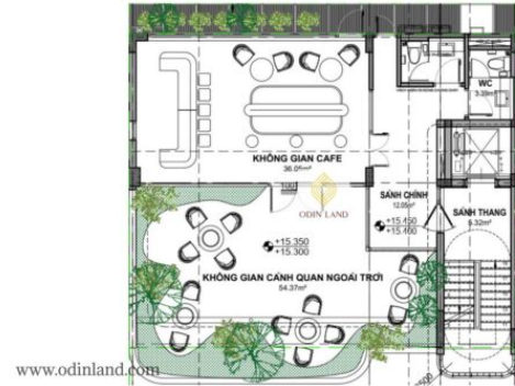
Sơ đồ mặt bằng tầng 4
