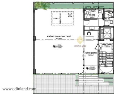
Sơ đồ mặt bằng tầng 1
