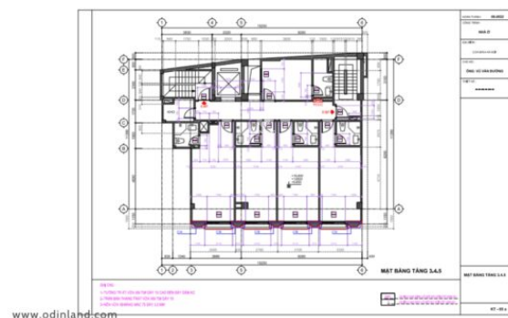
Mặt bằng tầng 3,4,5
