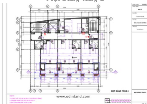
Mặt bằng tầng 6
