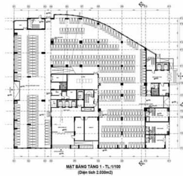
Sơ đồ mặt bằng
