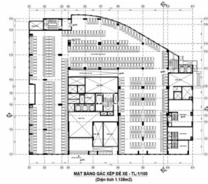
Sơ đồ mặt bằng
