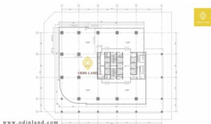
Sơ đồ mặt bằng tầng 05-17, 19-22
