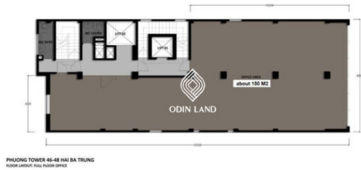
Sơ đồ mặt bằng các tầng tòa nhà Phuong Tower
