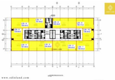
Sơ đồ mặt bằng tầng 29-30-33-34-37-38
