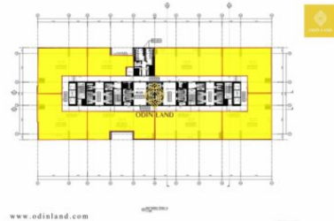
Sơ đồ mặt bằng tầng 14
