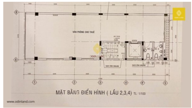
Sơ đồ mặt bằng tầng 2-4
