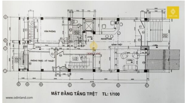
Sơ đồ mặt bằng tầng trệt
