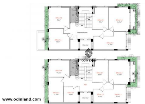
Sơ đồ mặt bằng tầng 1 và tầng 2
