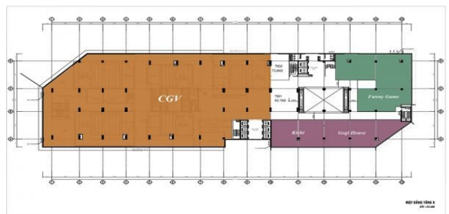
Sơ đồ mặt bằng tòa Artemis tầng 6
