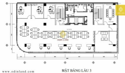
Sơ đồ mặt bằng tầng 3
