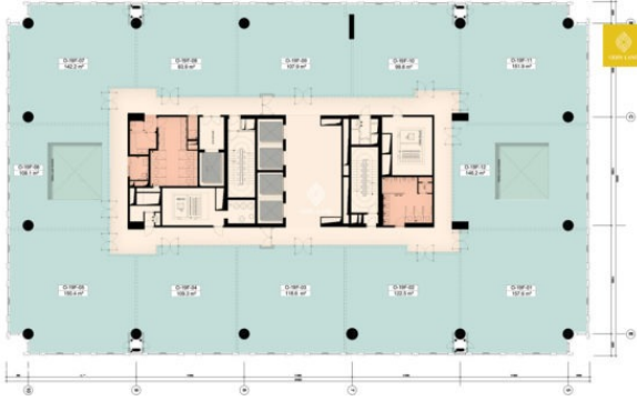
Sơ đồ mặt bằng tầng 19-21
