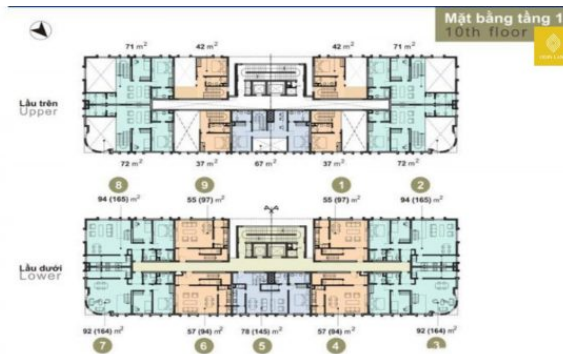
Sơ đồ mặt bằng tầng 10
