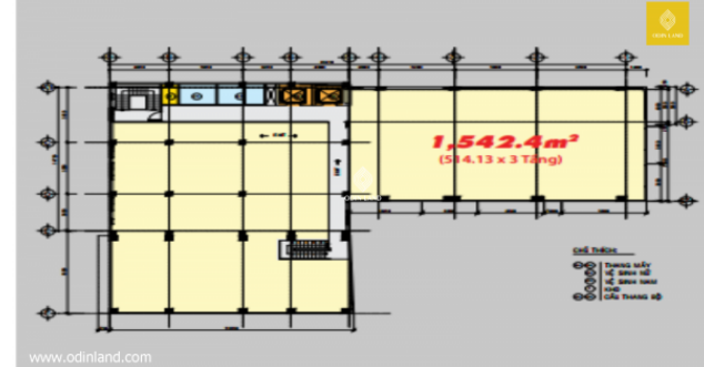
Sơ đồ mặt bằng tầng 2-4
