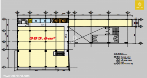
Sơ đồ mặt bằng tầng 1
