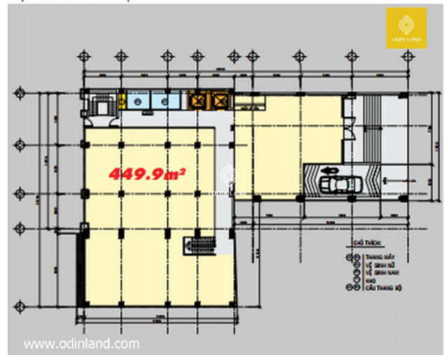
Sơ đồ mặt bằng tầng trệt
