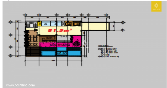
Sơ đồ Mặt Bằng Tầng 9
