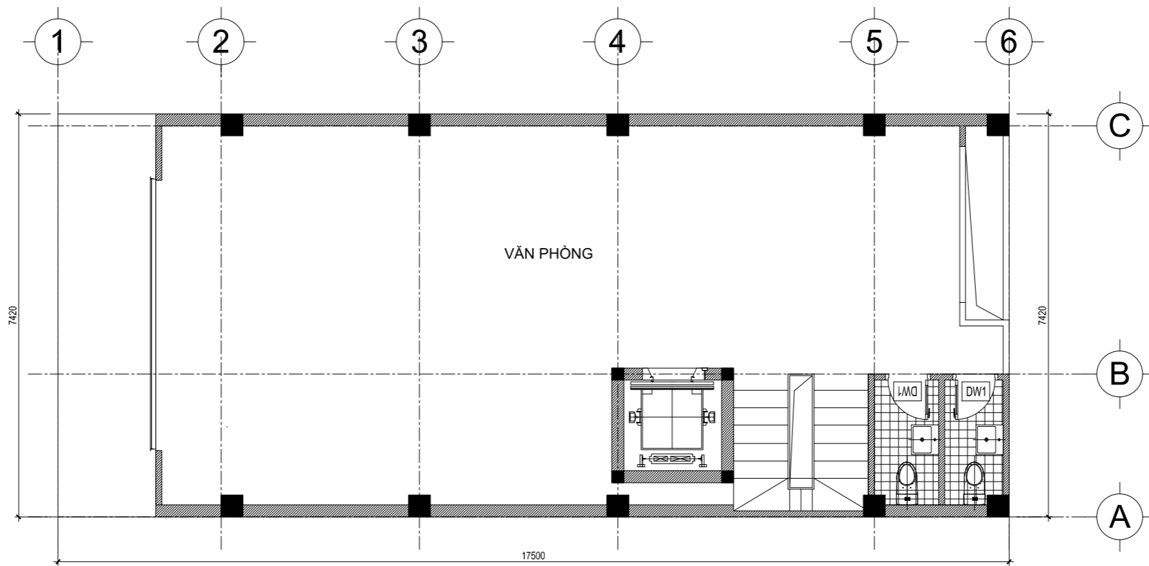
MẶT BẰNG TẦNG 2.3.4.5.6.7
